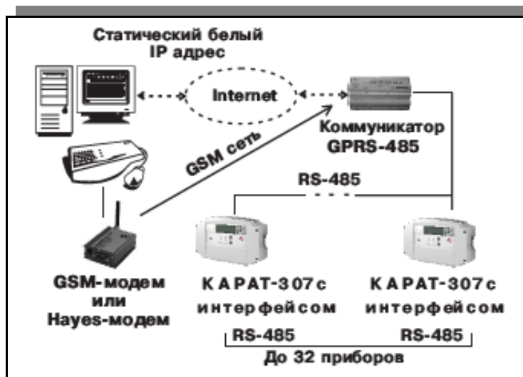
Рисунок 1.8 — Организация канала связи в режиме GPRS вариант 1
